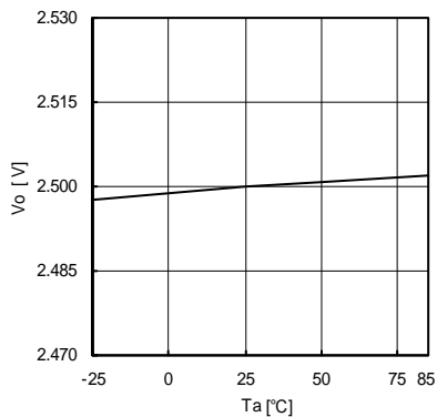
Fig.8 Ta-VO (IO=0A)
