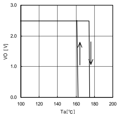
Fig.19 TSD (IO=0A)
