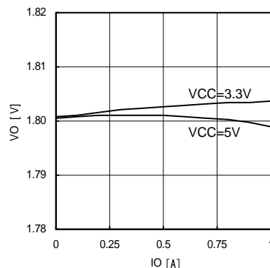
Fig.15 IO-VO (VO=1.8V)
