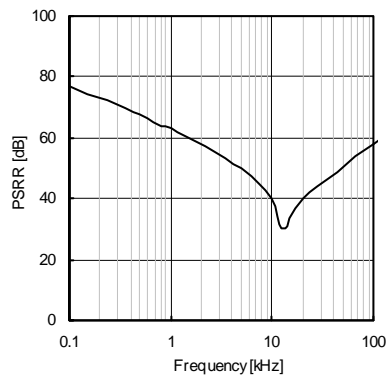
Fig.31 PSRR(IO=0A)
