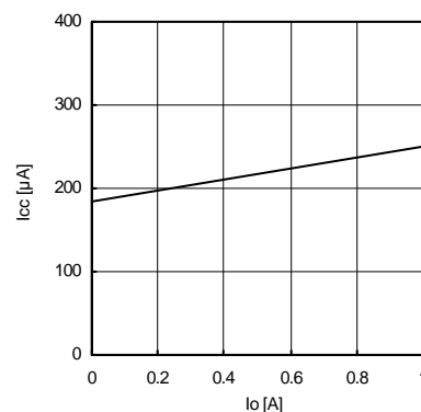
Fig.30 IO-ICC
