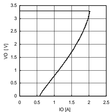
Fig.20 OCP (VCC=5V, VO=3.3V)
