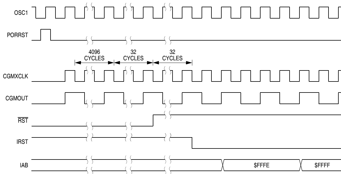
Figure 14-7. POR Recovery
