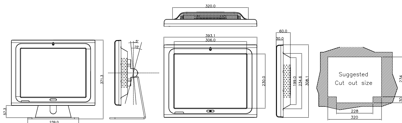
AFL-15A-N270
