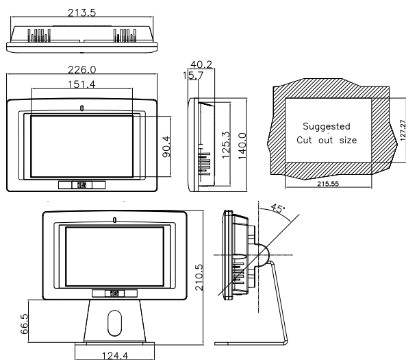
AFL-07A-N270
