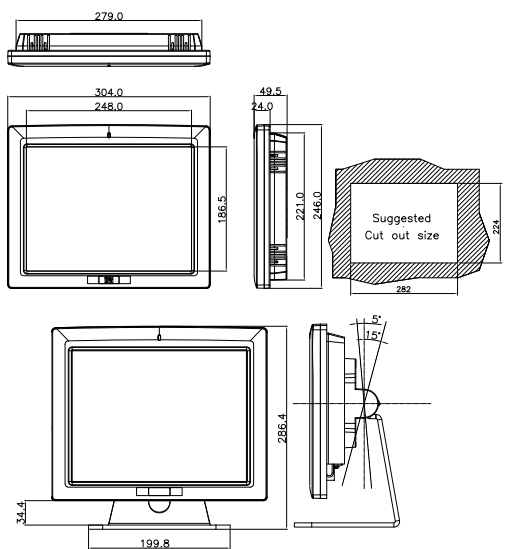
AFL-12A-N270
