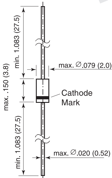
DO-204AH (DO-35)
