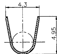
SECT A-A
