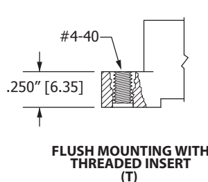
FLUSH MOUNTING (D)
