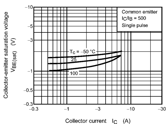
Fig. 7.6 V_{BE(sat)} - I_C
