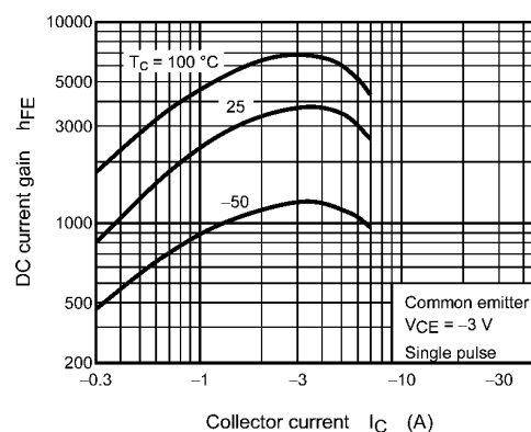
Fig. 7.4 h_{FE} - I_C
