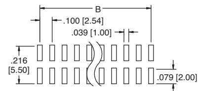
PH2-20-UA-SMT
