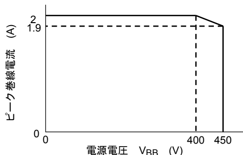
図 1: T_j = 135\text{ }^{\circ}\text{C} の安全動作領域
