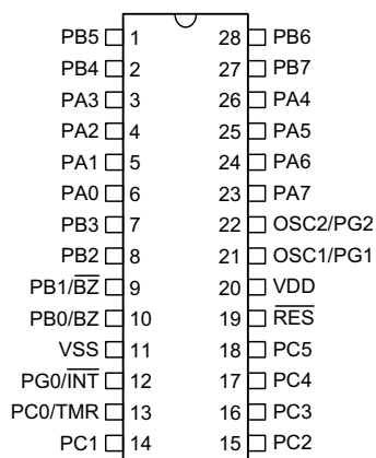
HT48R30A-1-A – 28 SKDIP/SOP
