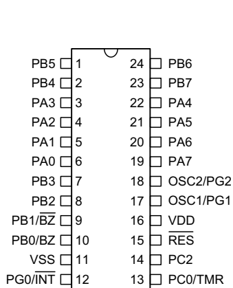
HT48R30A-1-A – 24 SKDIP/SOP
