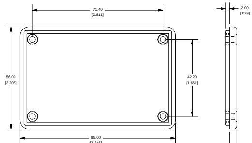
BOTTOM OF LID
