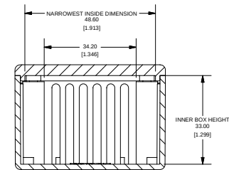
SECTION D-D SCALE 1 : 1
