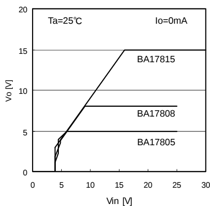
Fig.13 電源電圧－出力電圧 ( I_o=0\text{mA} )
