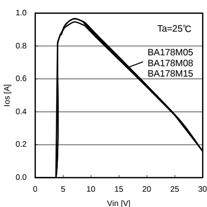
Fig.8 電源電圧－出力短絡電流
