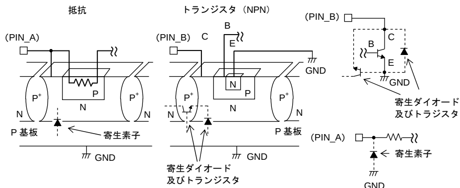
Fig.28 バイポーラ IC の簡易構造例
