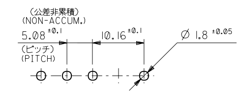
基板取付穴推奨寸法 RECOMMENDED P.C.B.HOLE DIMENSION
