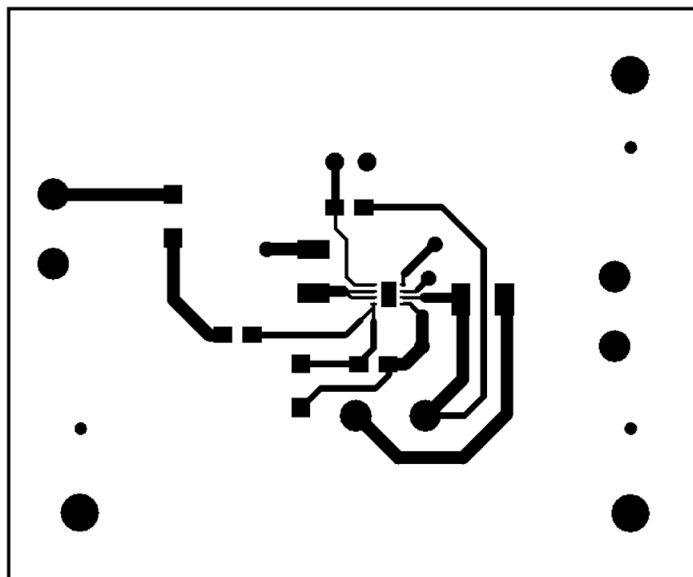
Figure 37. Top Layer
