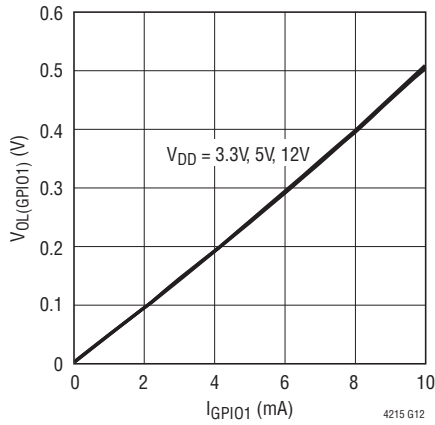
V_{OL}(\text{GPIO1}) vs I_{\text{GPIO1}}
