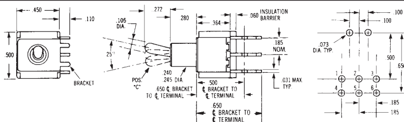
Right Angle P.C. Terminal
