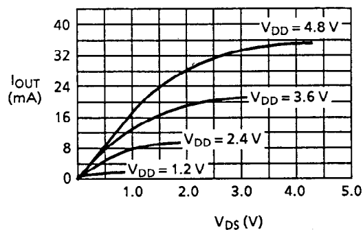
V_{DS} - I_{OUT}
