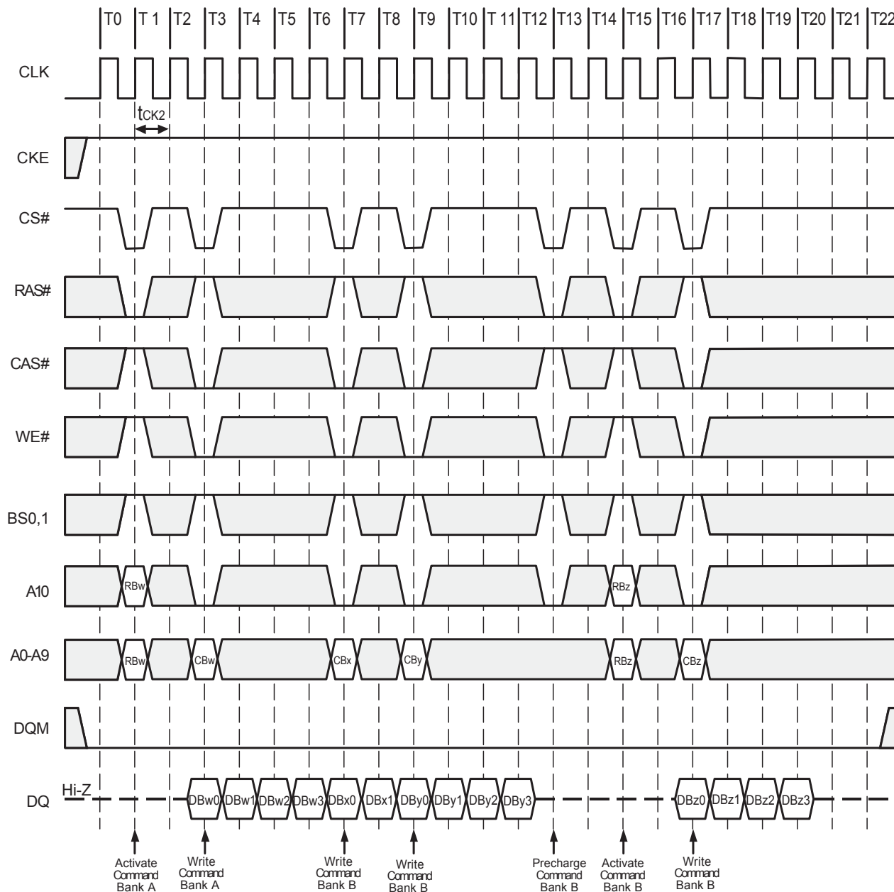
(Burst Length=4,CAS#Latency=2)
