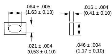
SOLDER LUG TERMINAL DETAIL 22.5°
