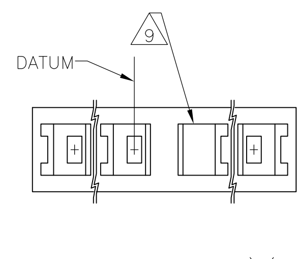
DETAIL Y
