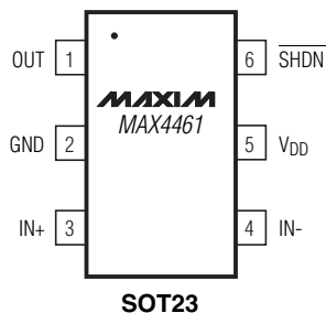
SOT23
