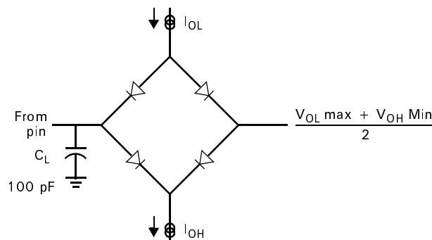
Figure 19. AC Parameter Test Circuit
