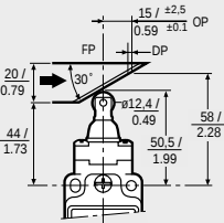
Top roller plunger
