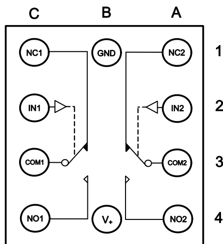
WLCSP-2.0×1.5-10B
