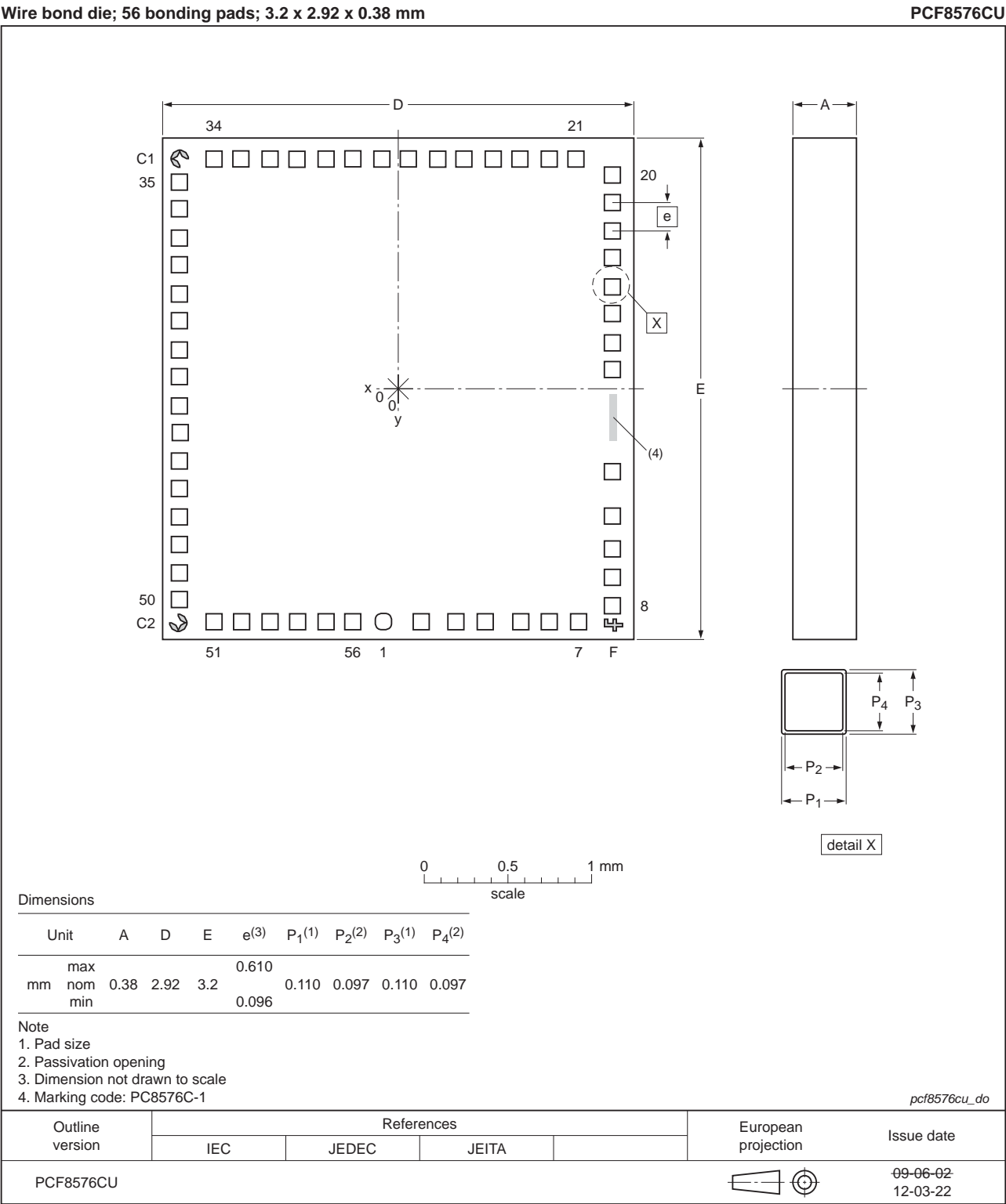
Fig 35. Bare die outline of PCF8576CU/F1
