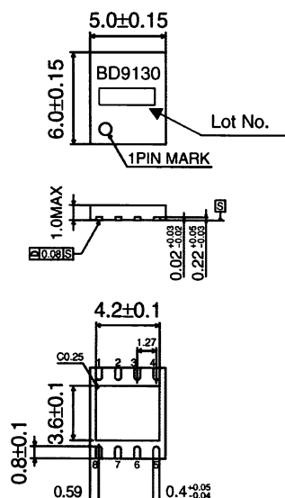
SON08V5060 (unit:mm)
