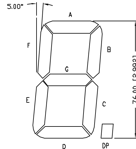
DIGIT DETAIL
