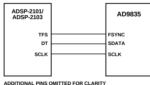
Figure 24. ADSP-2101/ADSP-2103-to-AD9835 Interface
