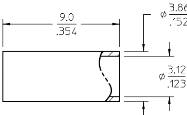
FERRULE
