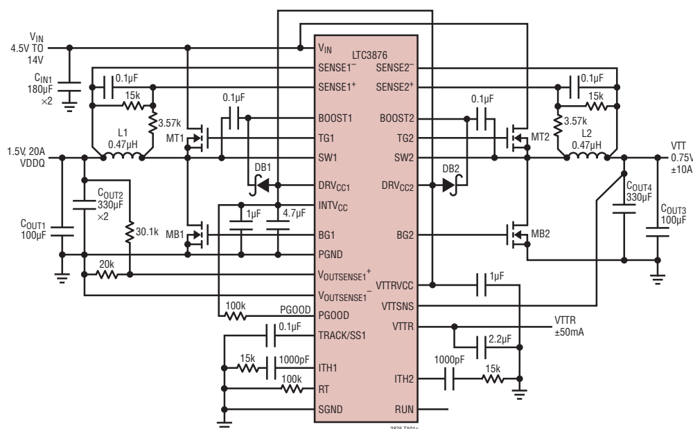
DDR3 1.5V VDDQ/20A 0.75VTT/±10A 4.5V to 14V Input
