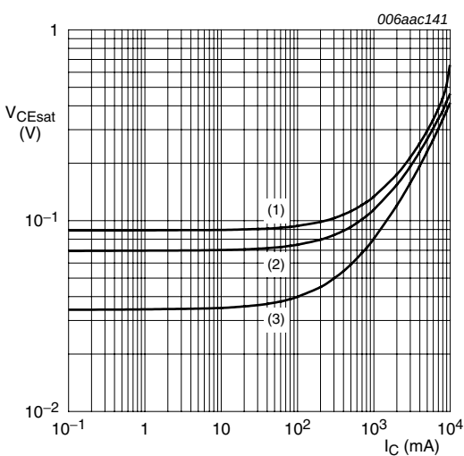
T_{amb} = 25\text{ }^{\circ}\text{C} (1) I_C/I_B = 100 (2) I_C/I_B = 50 (3) I_C/I_B = 10
