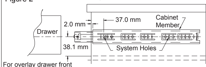
Figure 2 32 mm System—Cabinet
