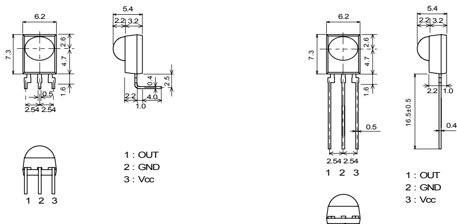
NJL21H000A UNIT:mm
