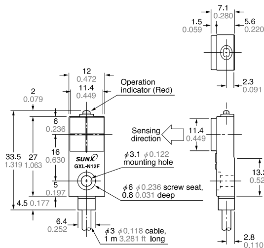
GXL-N12F type Sensor
