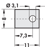
SOT 32
