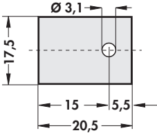
TOP 3/1
