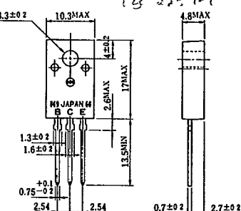
外形図 Outline Dimensions
