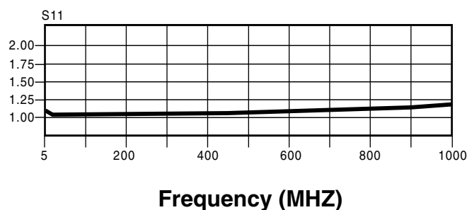
INPUT VSWR
