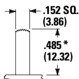
S6 0.485" High
