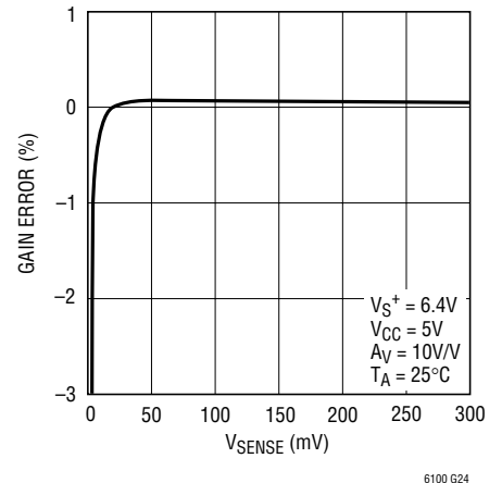
Gain Error vs VSENSE
