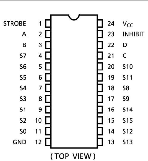
P (DIP24-P-300-2.54) Weight : 1.50g (Typ.)
