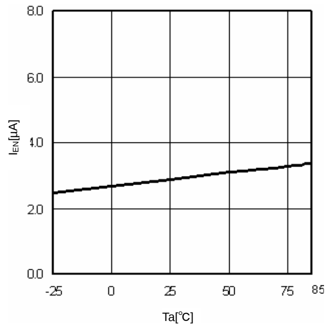
Fig.12 T_a - I_{EN}
