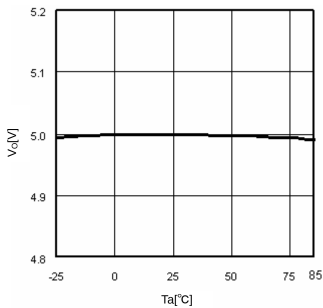
Fig.9 T_a-V_O ( I_O=0mA )
