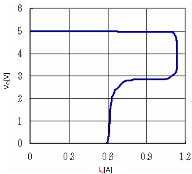
Fig.17 OCP
