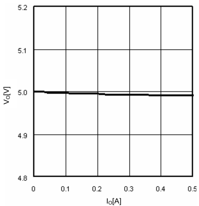
Fig.13 I_o - V_o
