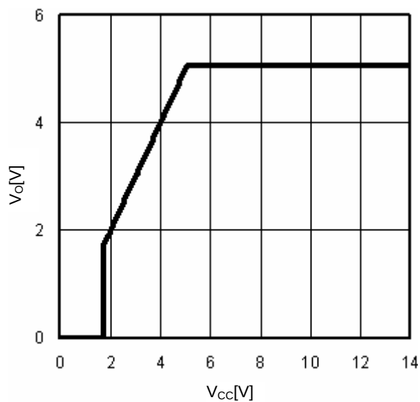
Fig.15 V_{CC}-V_O ( I_O=0\text{mA} )
