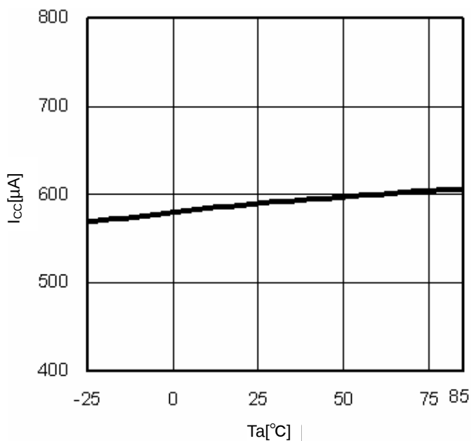
Fig.10 T_a-I_{cc}
