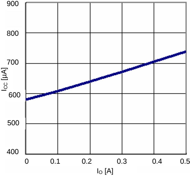
Fig.20 I_o - I_{cc}
