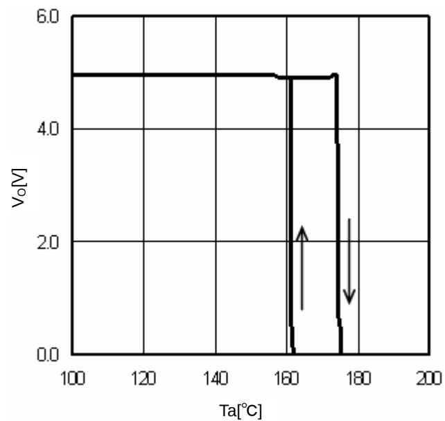
Fig.16 TSD ( I_O=0\text{mA} )
