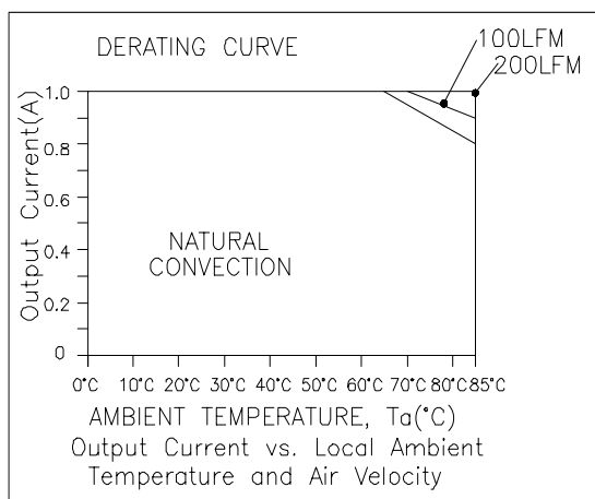
V_o=12\text{ V} , I_o=1\text{ A}
