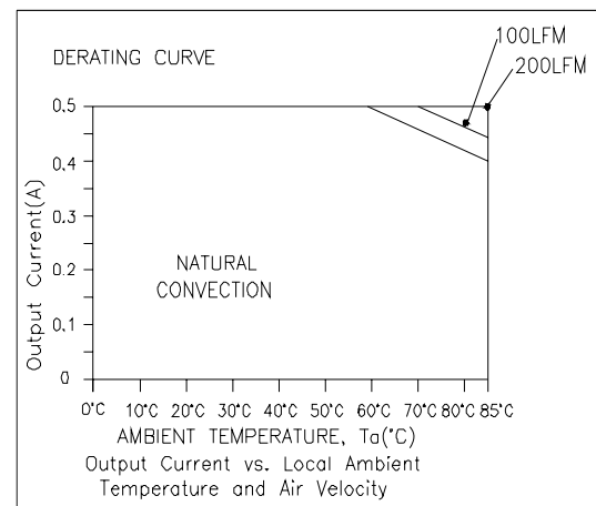
V_o=24\text{ V} , I_o=0.5\text{ A}
