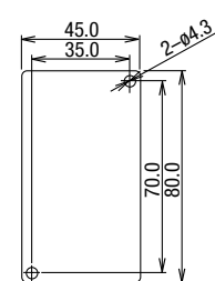
FC4A-SX5ES1E
