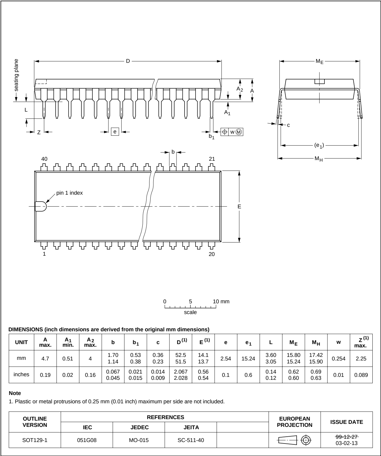
Fig 27. DIP40 (SOT129-1).
