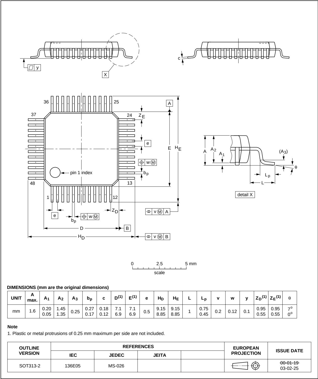
Fig 26. LQFP48 (SOT313-2).
