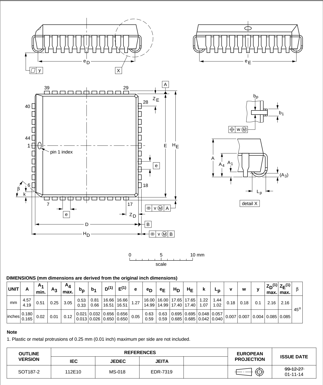
Fig 25. PLCC44 (SOT187-2).
