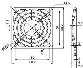
PB-06 For 60mm Fan
