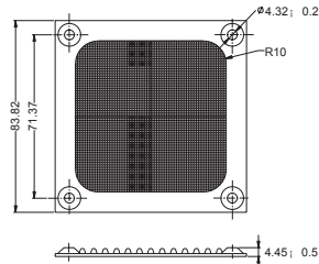
FM 08 For 80mm Fan
