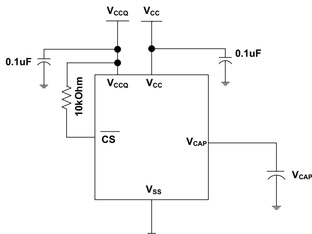
Figure 2. AutoStore Mode
